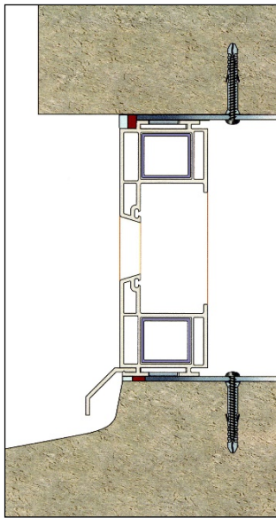
شکل ۱۲-۴۳- نصب غیر مستقیم پنجره و در به دیوار توپر بنایی یا بتنی توسط بست و رول پلاگ
