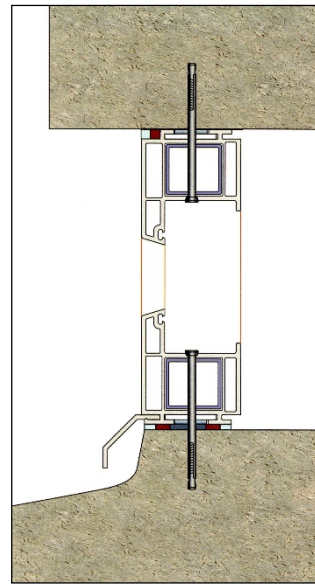
شکل ۱۲-۴۲- نصب مستقیم پنجره و در به دیوار توپر بنایی یا بتنی توسط رول بولت
