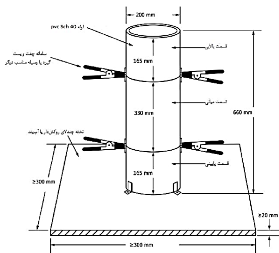
شکل ۸-۳ دستگاه ستون جدادگی ایستایی مطابق استاندارد ملی ایران ۱۲۲۵۵
