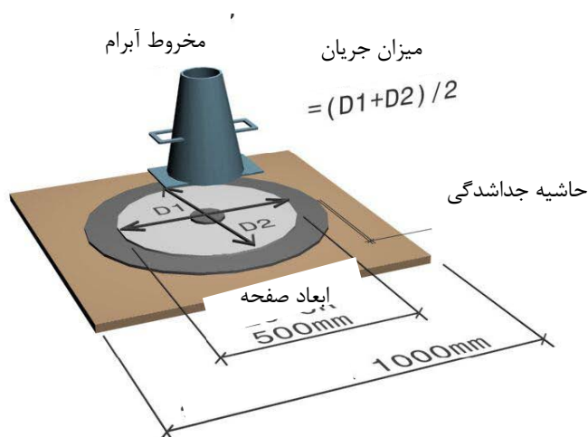
شکل ۱-۳ مشخصات ابزار و وسایل اندازه‌گیری جریان اسلامپ
