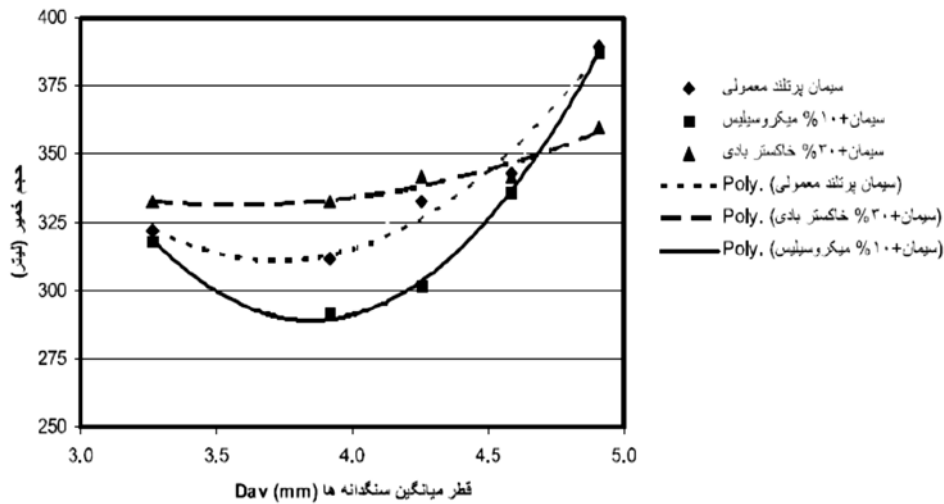
شکل ۲-۴ حداقل حجم خمیر سیمان لازم
